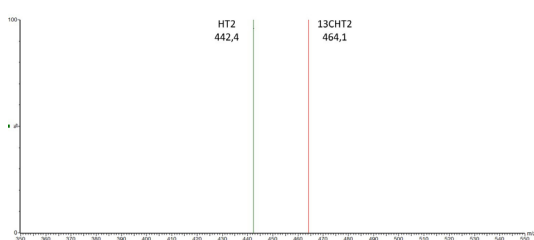
Spectre MS de la Toxine HT2 et étalon LIB'UP® U-[ 13 C22]-Toxine HT2
